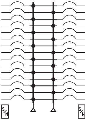
125–250 A Main Lugs
